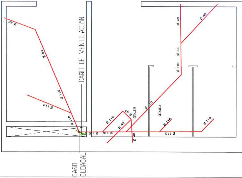
PLANTA ISOMETRIA DE AGUAS CLOACALES ALA NORTE
