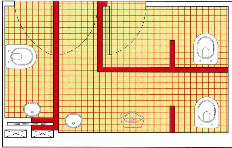
PLANTA DEMOLICIÓN ALA NORTE
