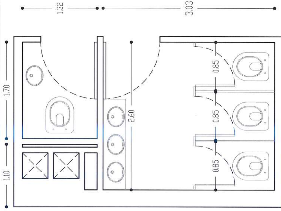
PLANTA DISTRIBUCIÓN DE BAÑOS ALA SUR
