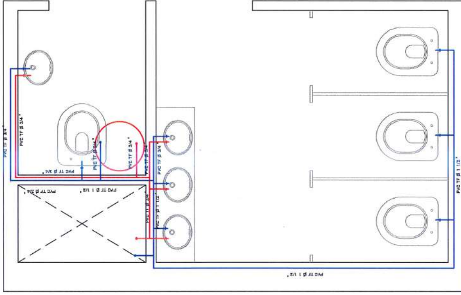
PLANTA DE INSTALACIONES DE AGUA FRIA Y AGUA CALIENTE ALA SUR
