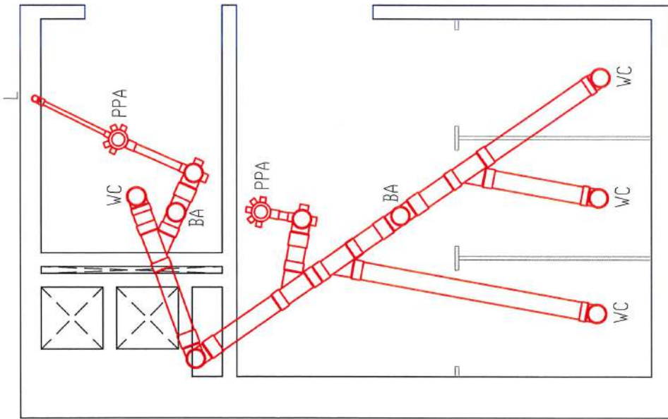
DETALLE C - PLANTA DE DESAGÜES CLOACALES ALA SUR
