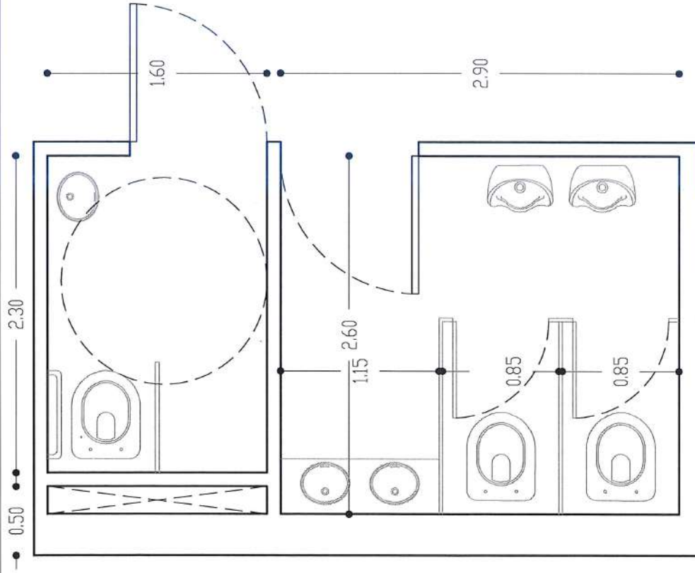
PLANTA DISTRIBUCIÓN DE BAÑOS ALA NORTE
