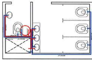
PLANTA DE INSTALACIONES DE AGUA FRIA Y AGUA CALIENTE ALA SUR
