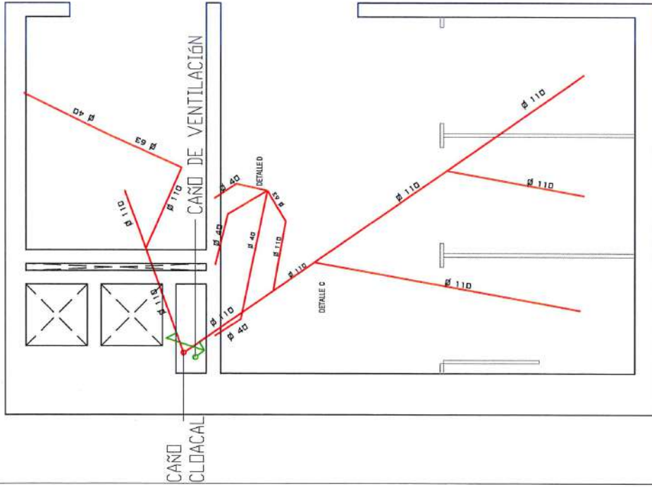
PLANTA ISOMETRÍA DE AGUAS CLOACALES ALA SUR
