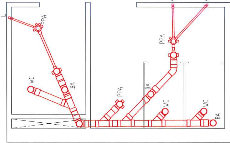
DETALLE A - PLANTA DE DESAGUES CLOACALES ALA NORTE
