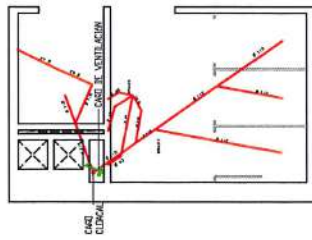
PLANTA DISTRIBUCIÓN DE AGUAS CLOACALES ALA SUR
