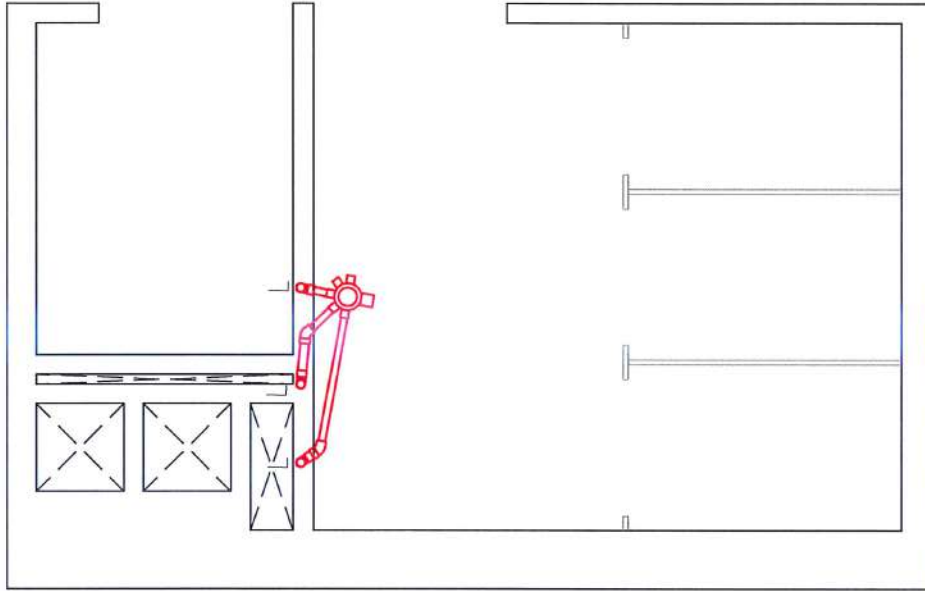
DETALLE D - PLANTA DE DESAGÜES CLOACALES ALA SUR
