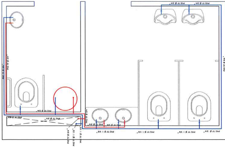
PLANTA DE INSTALACIONES DE AGUA FRIA Y AGUA CALIENTE ALA NORTE
