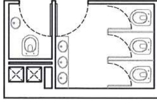
PLANTA DISTRIBUCION DE AGUAS FRIA SUR
